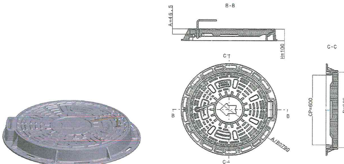
CAPAC C600 CLASA C250
